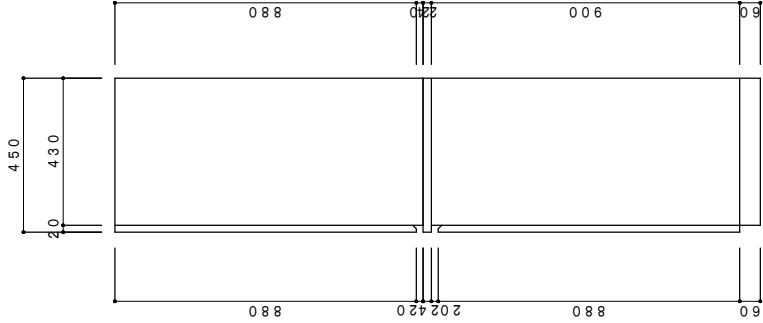
側面立面図 1/15
