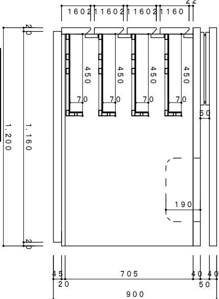
側面断面図 1/15
