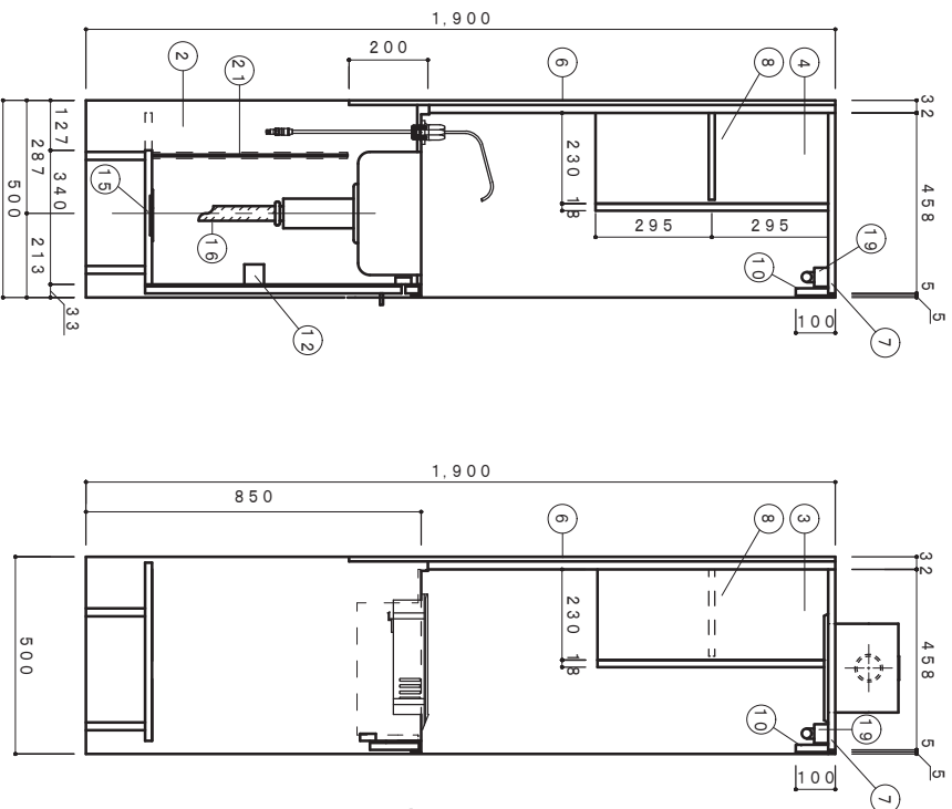
側面断面図 1/15
