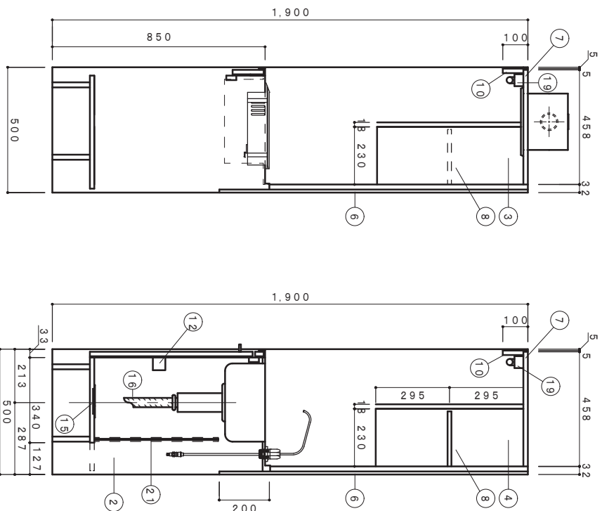
側面断面図 1/15
