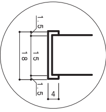
A部詳細図
