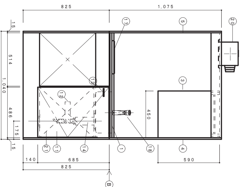
正面図 1/15
