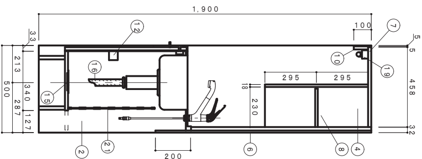
側面断面図 1/15
