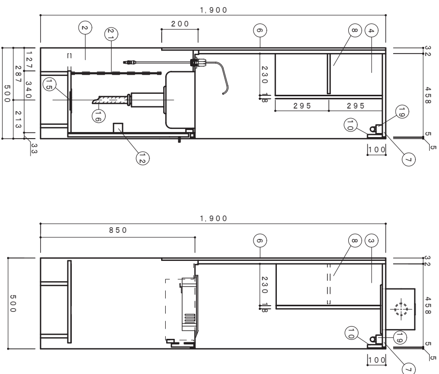
側面断面図 1/15
