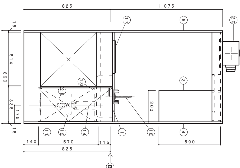
正面図 1/15
