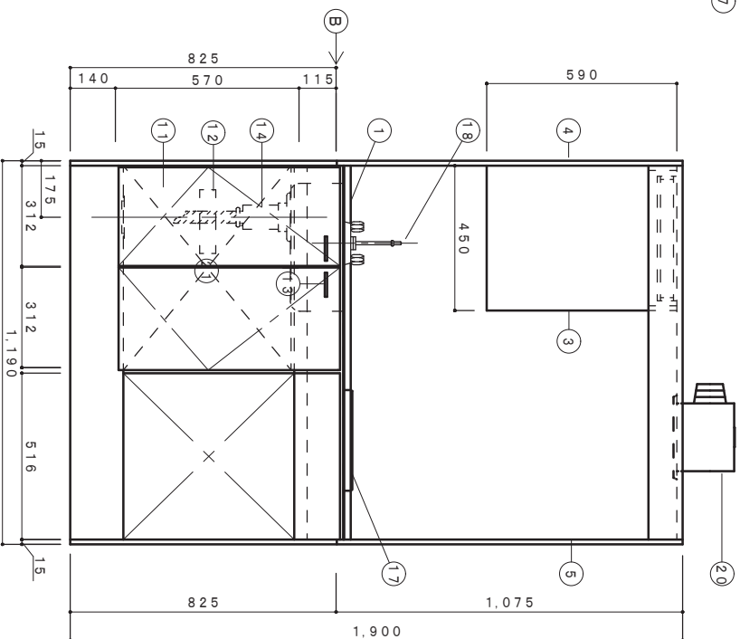
正面図 1/15
