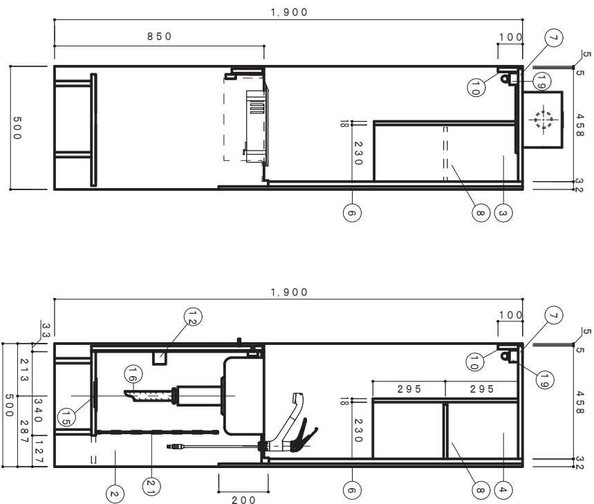
側面断面図 1/15
