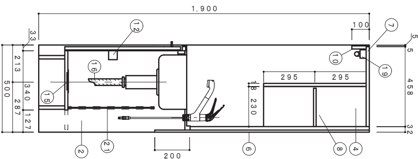
側面断面図 1/15
