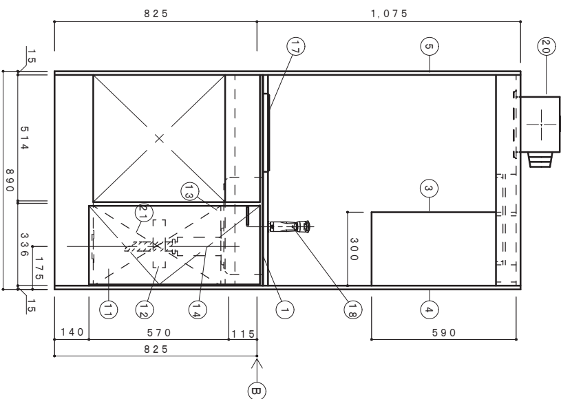
正面図 1/15
