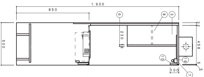
側面断面図 1/15
