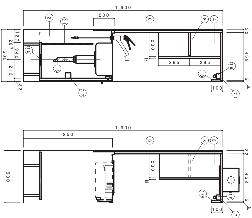
側面断面図 1/15
