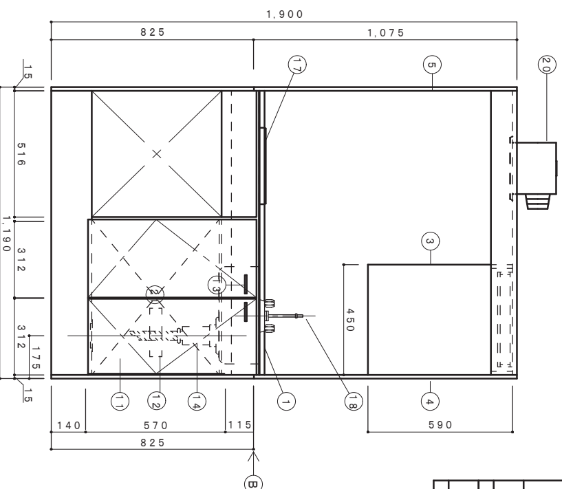
正面図 1/15
