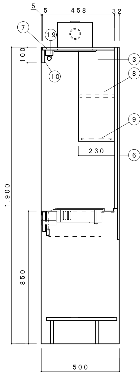
側面断面図 1/15
