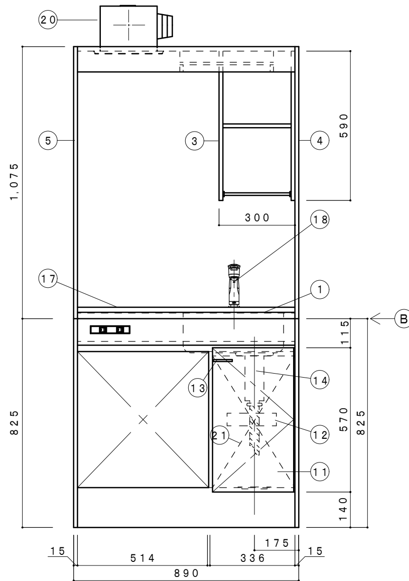
正面図 1/15
