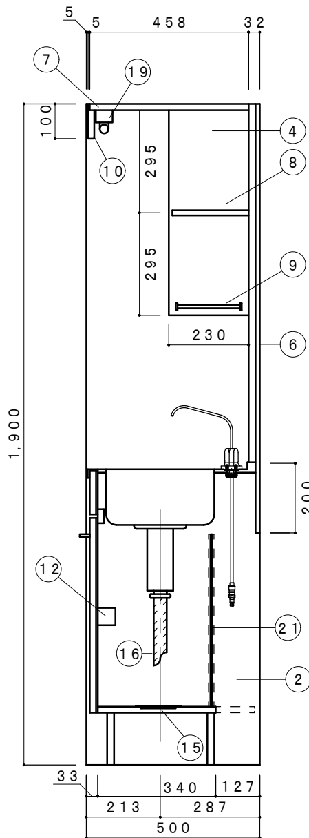
側面断面図 1/15
