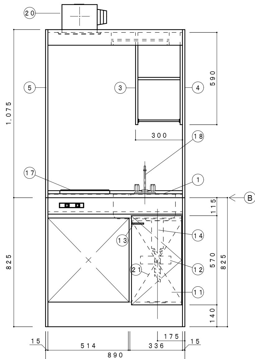
正面図 1/15
