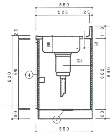
側面断面図 1/15
