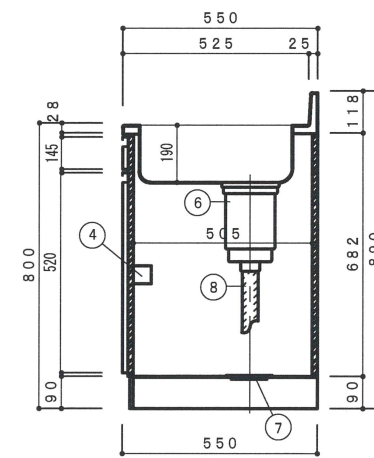
側面断面図 1/15
