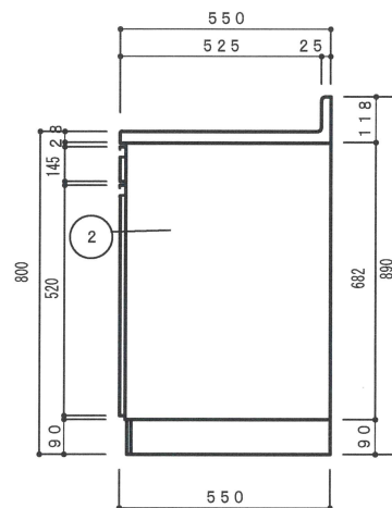
側面立面図 1/15
