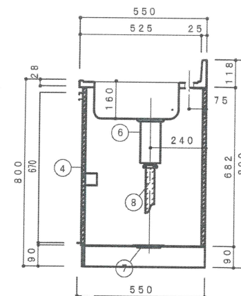
側面断面図 1/15
