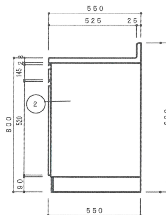
側面立面図 1/15
