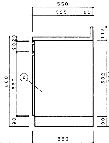
側面立面図 1/15
