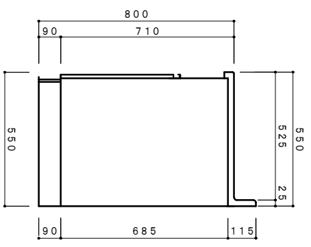
側面立面図 1/15
