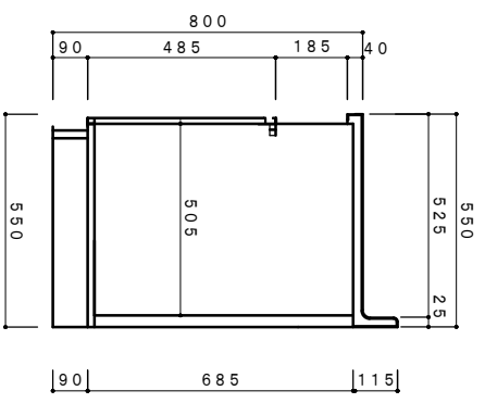
側面断面図 1/15
