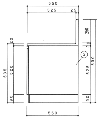
側面立面図 1/15
