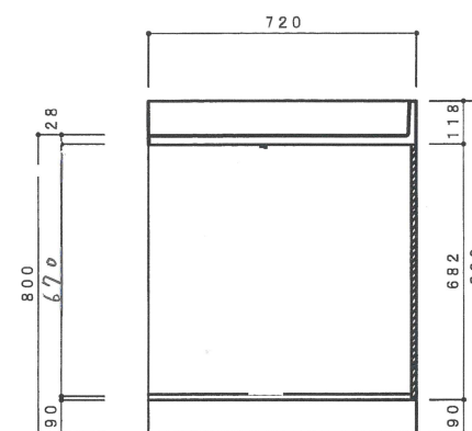
側面断面図 1/15
