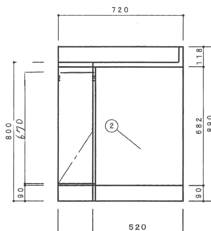
側面立面図 1/15
