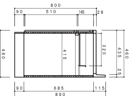
側面断面図 1/15
