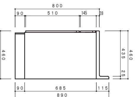
側面立面図 1/15
