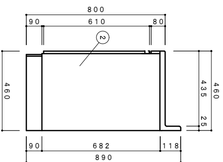
側面立面図 1/15
