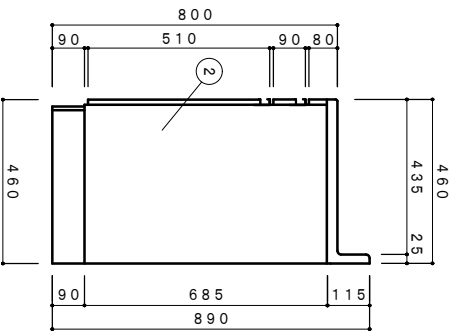
側面立面図 1/15
