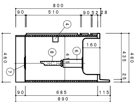
側面断面図 1/15
