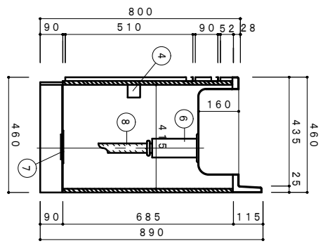
側面断面図 1/15
