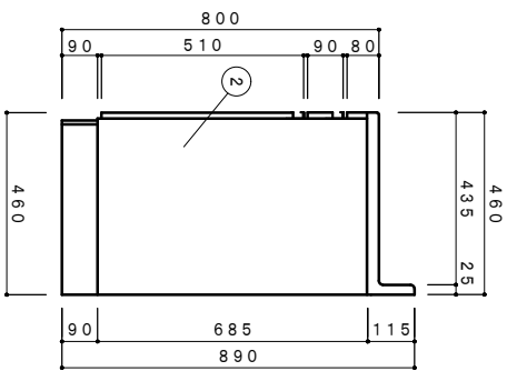
側面立面図 1/15
