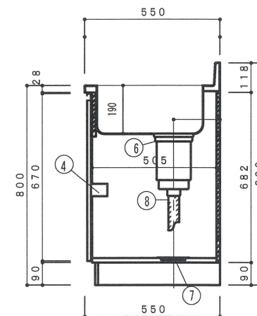
側面断面図 1/15
