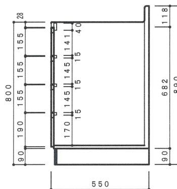
側面立面図 1/15
