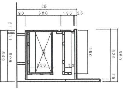
側面断面図 1/15
