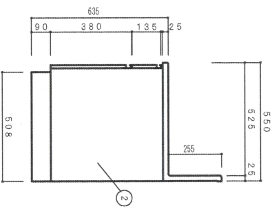
側面立面図 1/15
