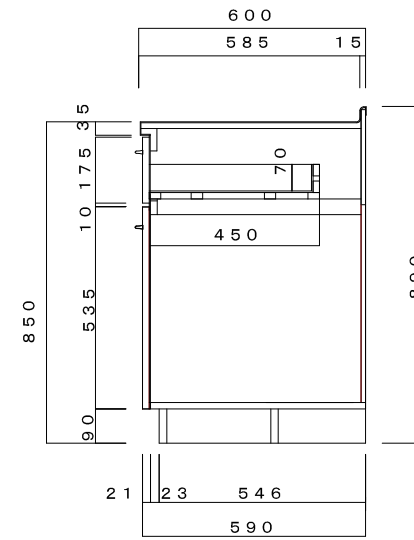
側面断面図 1/20
