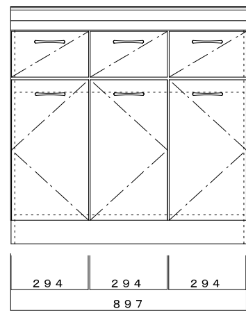
正面図 1/20
