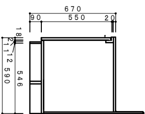
側面断面図 1/20
