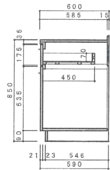
側面断面図 1/20
