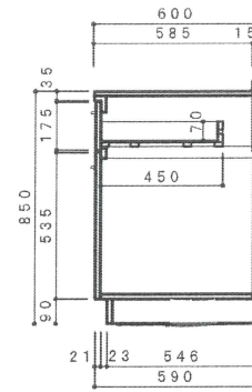
側面断面図 1/20
