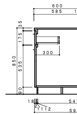
側面断面図 1/20
