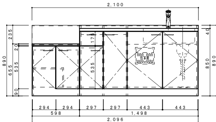
正面図 1/20
