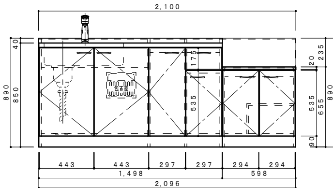
正面図 1/20
