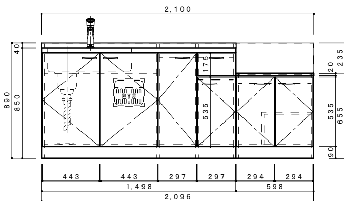
正面図 1/20
