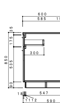
側面断面図 1/20
