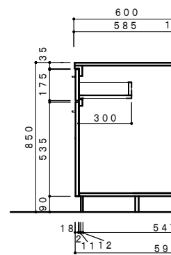
側面断面図 1/20
