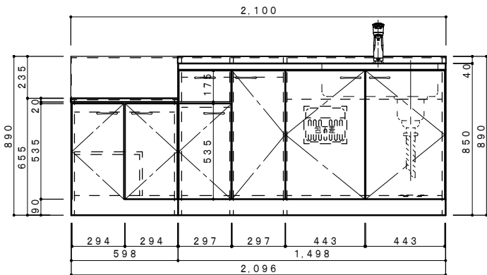
正面図 1/20
