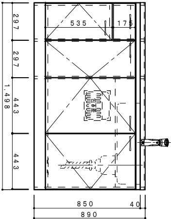
正面図 1/20
