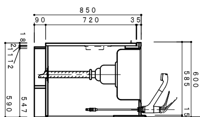
側面断面図 1/20
