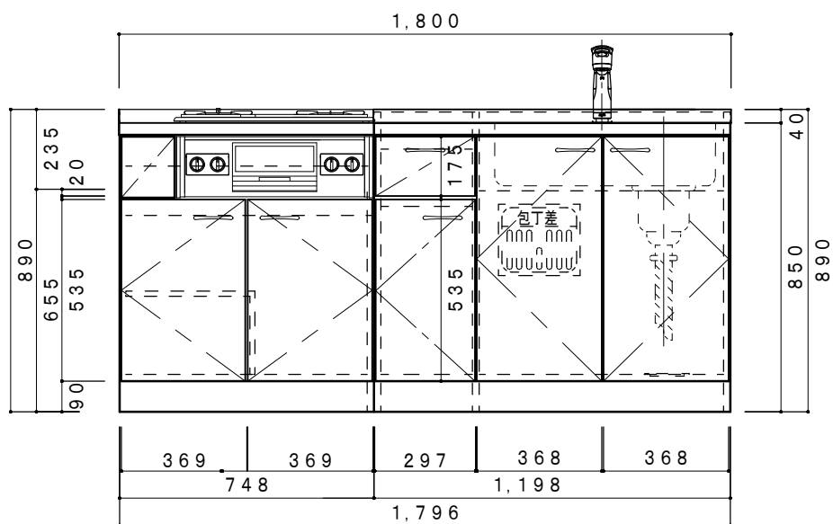
正面図 1/20
