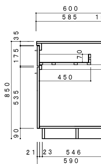
側面断面図 1/20
