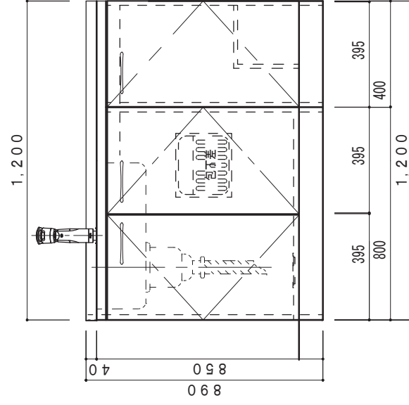
正面図 1/20
