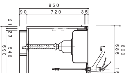
側面断面図 1/20
