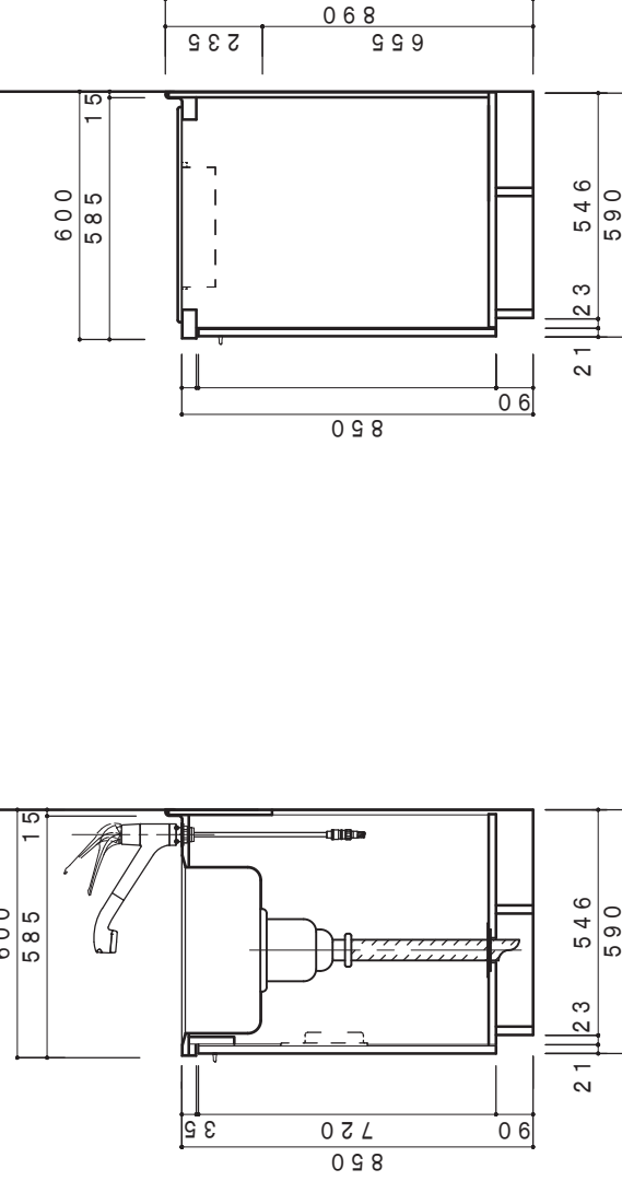
側面断面図 1/20
