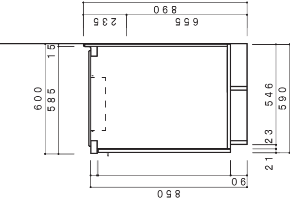
側面断面図 1/20
