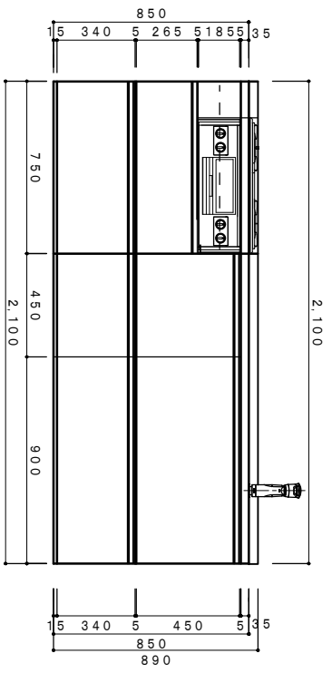
正面図 1/20
