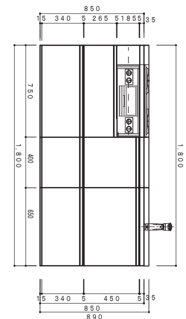
正面図 1/20
