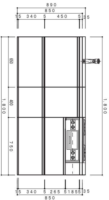
正面図 1/20
