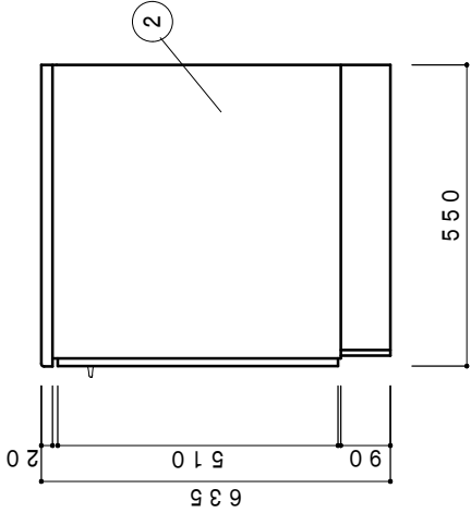
側面立面図 1/15
