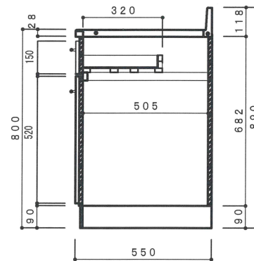
側面断面図 1/15
