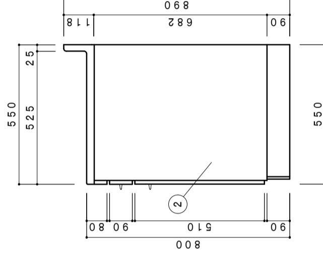
側面立面図 1/15
