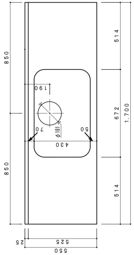
天板開口寸法図 1/15
