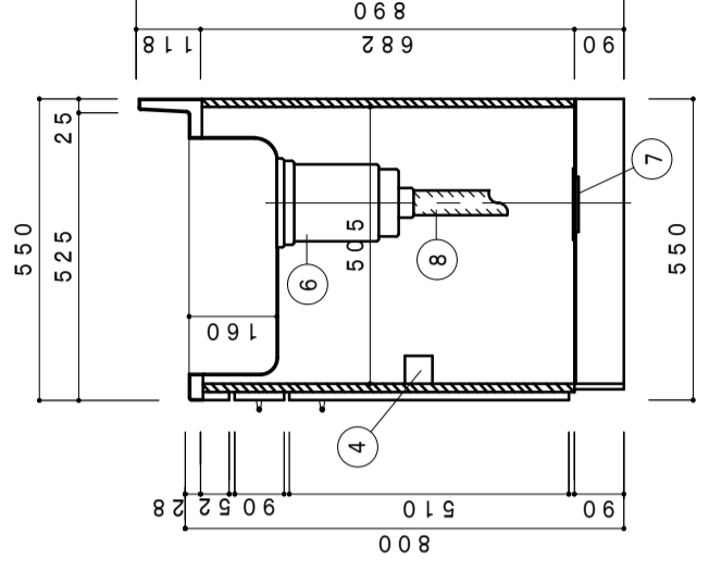
側面断面図 1/15
