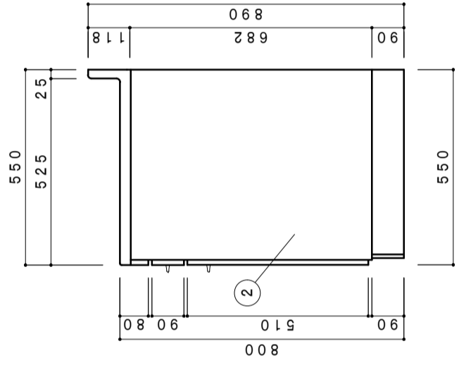
側面立面図 1/15
