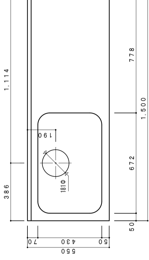
【天板開口寸法図 1/15】
