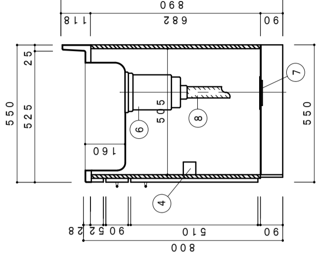
側面断面図 1/15
