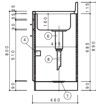
側面断面図 1/15
