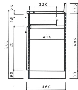
側面断面図 1/15
