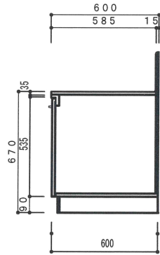
側面断面図 1/20
