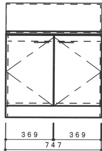
正面図 1/20
