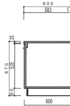
側面断面図 1/20
